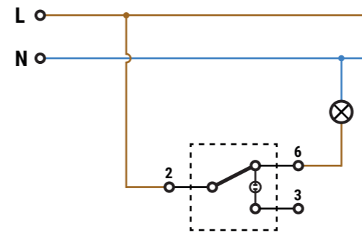
CONMUTADOR ERP02ILU
