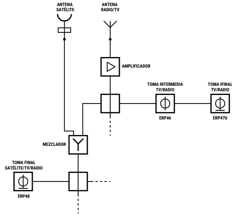
RADIO/TV/SATÉLITE ERP46/ERP47/ERP48
