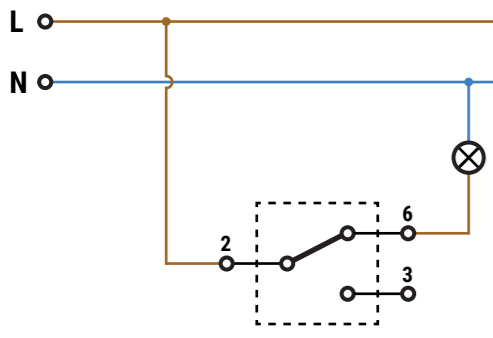
CONMUTADOR ERP02
