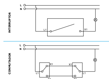
Conmutador/ Interruptor
