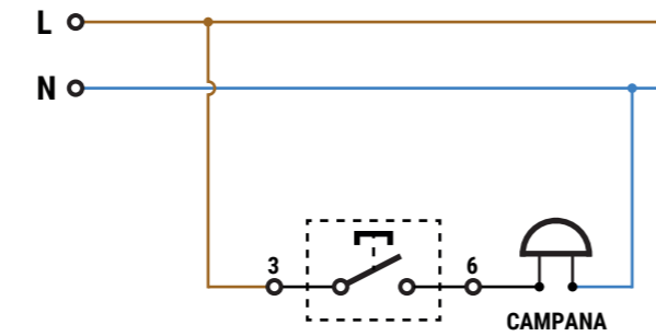
PULSADOR LUZ MUR04
