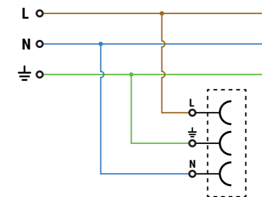
BASE FIJA 2P+T MUR60
