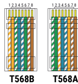
TOMA DE DATOS RJ45 MUR88/MUR87
