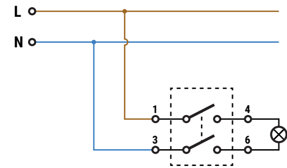
DOBLE INTERRUPTOR MUR12
