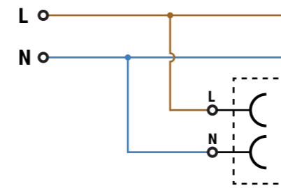
BASE FIJA 2P MUR07
