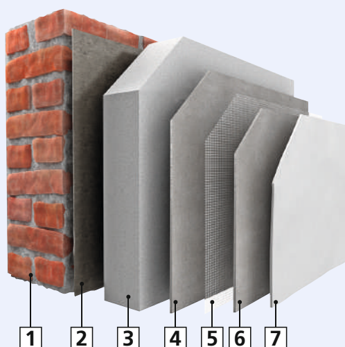
1 Mampostería | 2 Adherencia | 3 Placa aislante | 4 Revestimiento de refuerzo | 5 Tejido de refuerzo | 6 Revestimiento de refuerzo | 7 Revestimiento exterior
