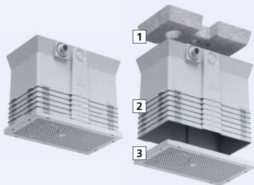
1 Elemento de aislamiento, 2 ThermoX® Iso +, 3 Panel frontal (N.º artículo 1159-70)
