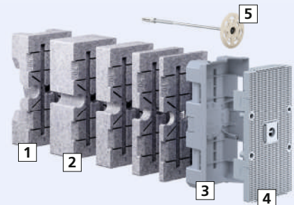
Portaequipos del sistema con placa de montaje universal N.º artículo 9966.21 / 22
