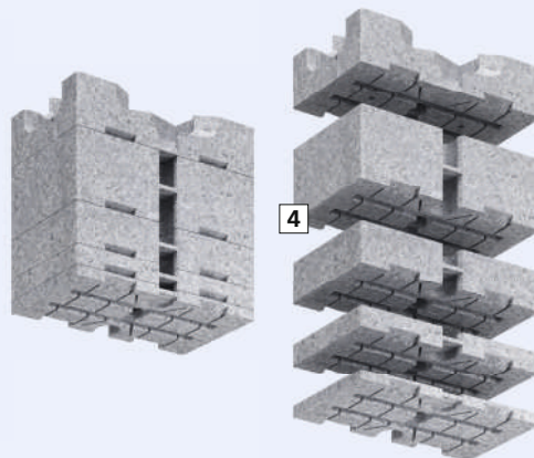
4 Elemento de extensión (N.º artículo 1159-71)
