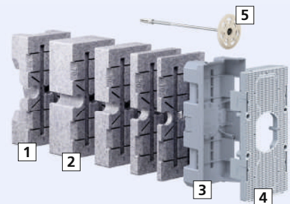
1 Elemento básico | 2 Elementos intermedios | 3 Base de la carcasa | 4 Panel frontal | 5 Clavija de tornillo
