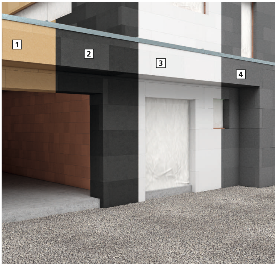
1 Aislamiento de fibra de madera | 2 Espuma de vidrio | 3 Espuma mineral | 4 EPS
